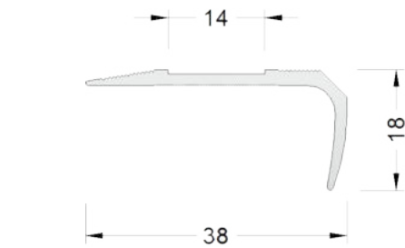
Treppenkantenprofil 38x18 ASM G, L=300cm
