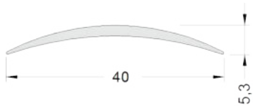
Nahtdeckprofil 40x2mm ASM G, L=270cm
