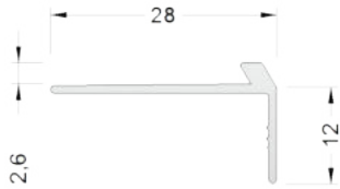
Treppenkantenprofil 28x12x2,6mm ASM G, L=300cm
