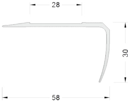
Treppenkantenprofil 58x30mm ASM G, L=300cm
