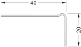
Reparaturwinkel Typ S für Beton, 30x1m
