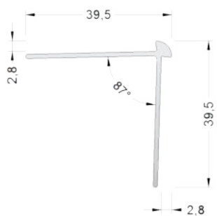
Treppenkantenprofil 2,8mm, ASM beidseitig G, L=300cm Treppenkantenprofil 2,8mm, Alu natur beidseitig G, L=300cm
