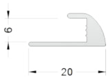
Abschlussprofil 6mm Alu silber matt G, L=270cm
