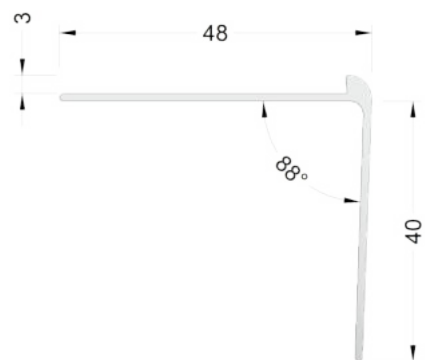
Treppenkantenprofil 40x48x3mm ASM G, L=300cm
