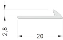
Abschlussprofil 2,8mm Alu silber matt G, L=270cm
