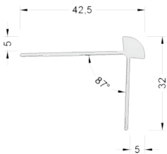
Treppenkantenprofil 5mm ASM einseitig G, L=300cm Treppenkantenprofil 5mm, Alu natur einseitig G, L=300cm
