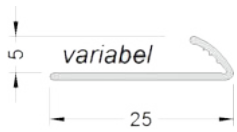
Abschlussprofil 5mm (leicht) Alu silber matt G, L=270cm
