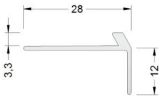
Treppenkantenprofil 28x12x3,36mm ASM G, L=300cm
